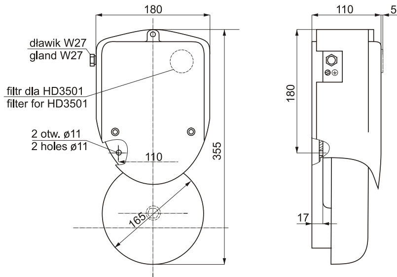
Rysunek gabarytowy Dimensioned drawing
