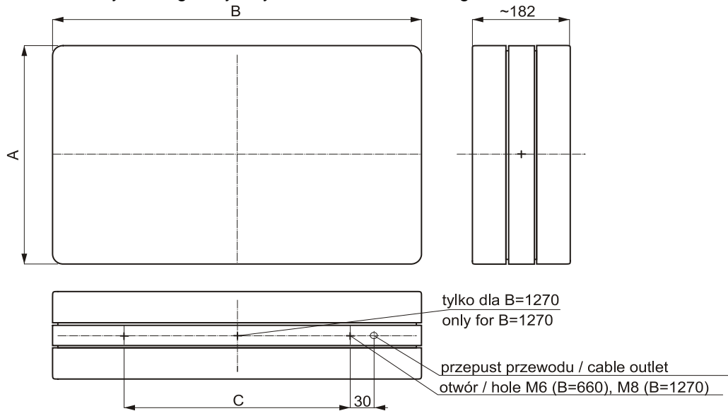
Rysunek gabarytowy / Dimensioned drawing
