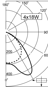
odbly nik paraboliczny / parabolic louvre
