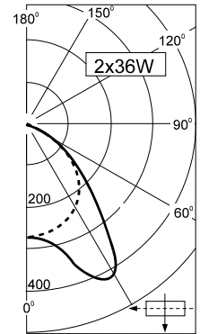
odbly nik paraboliczny / parabolic louvre
